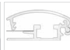
Profil ramy
